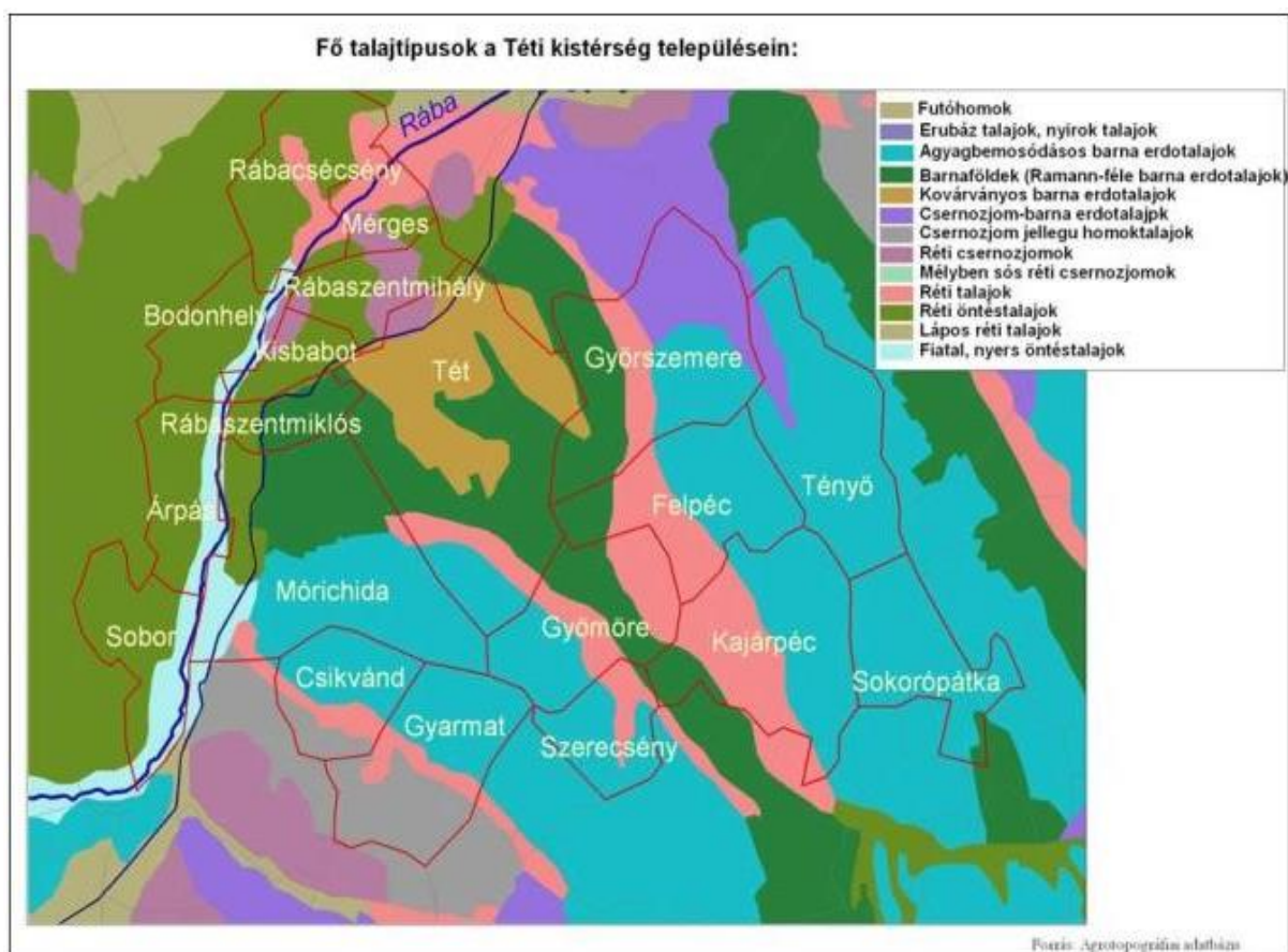
1-67. ábra: Fő talajtípusok a Téli járásban, forrás: A SOTT környezetvédelmi programjának felülvizsgálata
