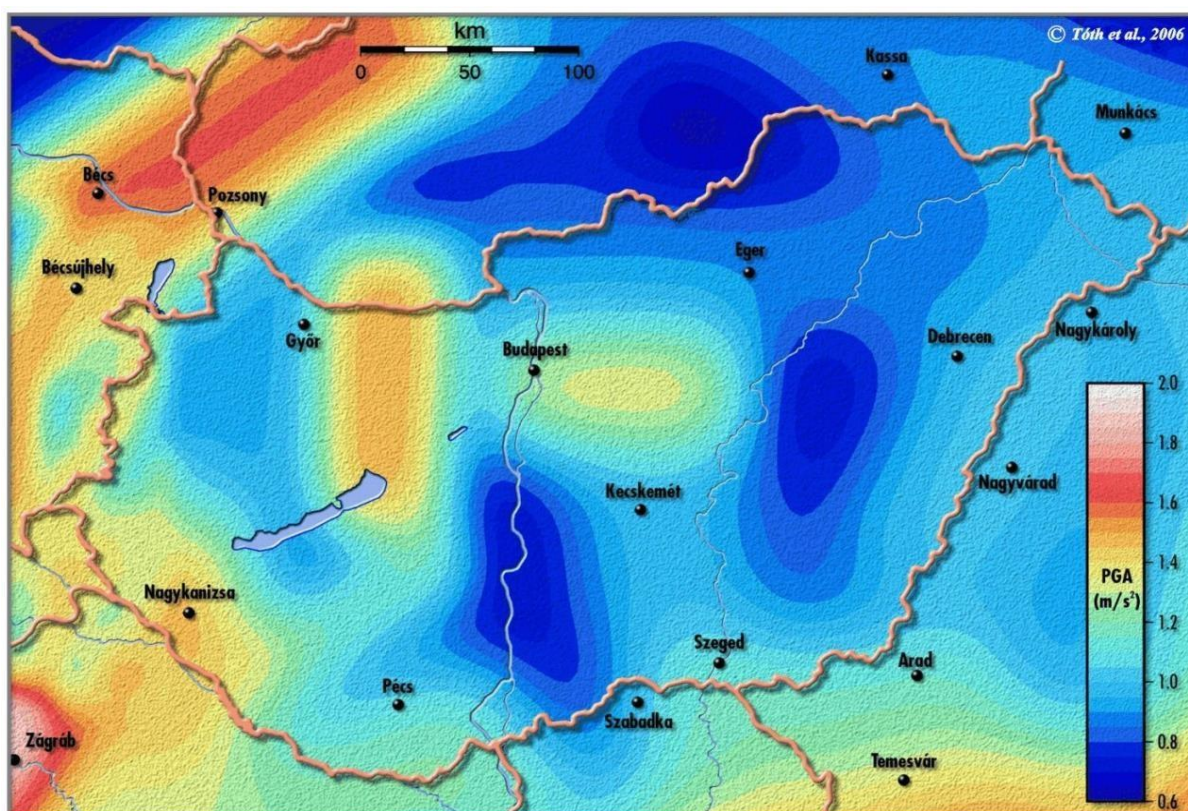
1-101. ábra: Magyarország földrengés-veszélyeztetettsége (Forrás: http://mkweb.uni-pannon.hu/tudastar/ff/10-vesz/images/001.png )
