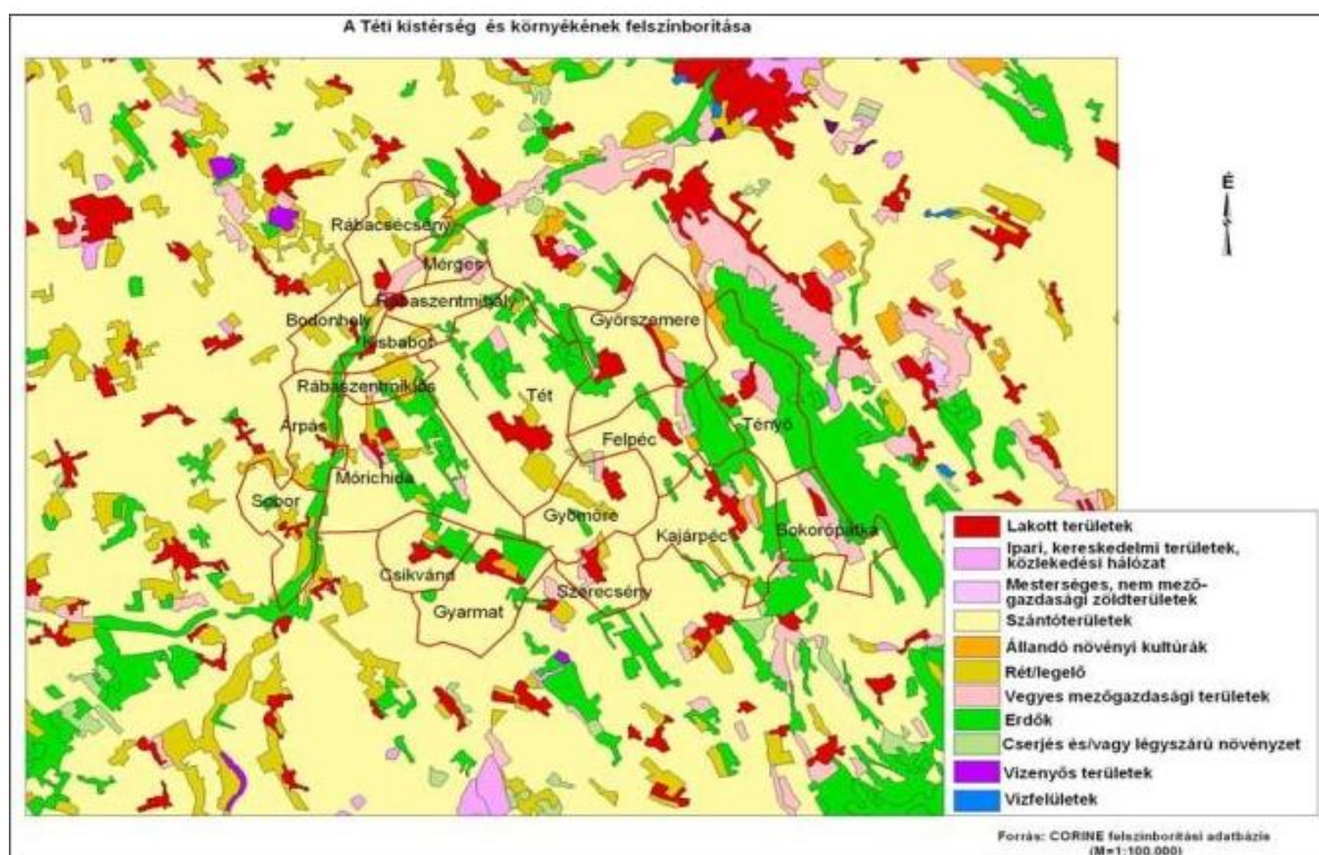
1-69. ábra: A Téti járás és környékének felszínborítottsága Forrás: A SOTT környezetvédelmi programjának felülvizsgálata
