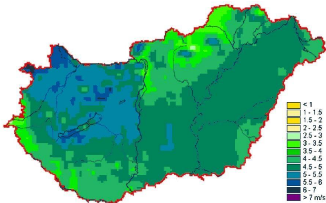
1-98. ábra: Országos energetikai széltérkép Forrás: Magyar Meteorológiai Szolgálat
