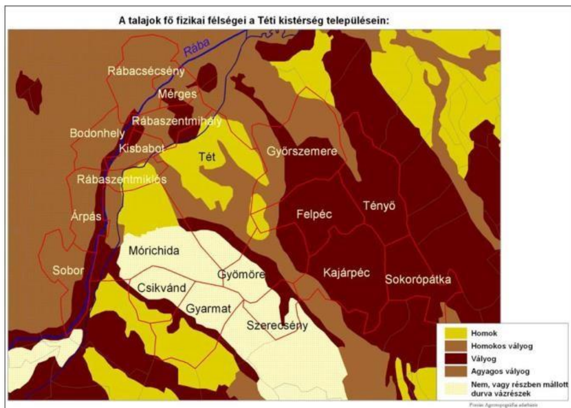
1-68. ábra: A talajok fő fizikai félségei a Téli-járásban, forrás: A SOTT környezetvédelmi programjának felülvizsgálata
