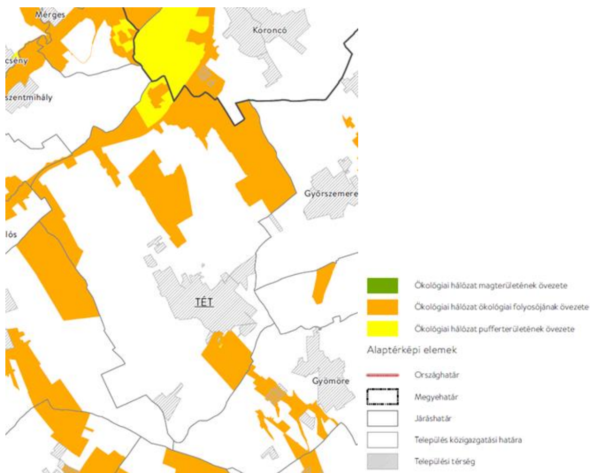
1-71. ábra: A Téti járás településeit érintő ökológiai hálózati elemek Forrás: Országos Területrendezési Terv
